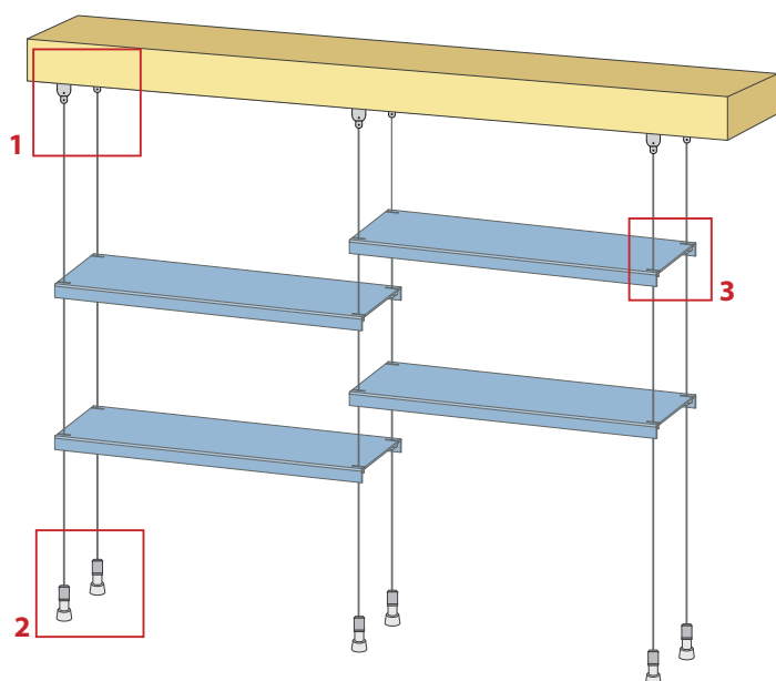
1. ANCORAGGIO FISSO
